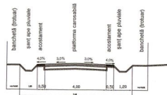
Secțiune caracteristică străzi reabilitate, 4,00 m
