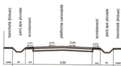
Secțiune caracteristică străzi reabilitate, 5,50 m
