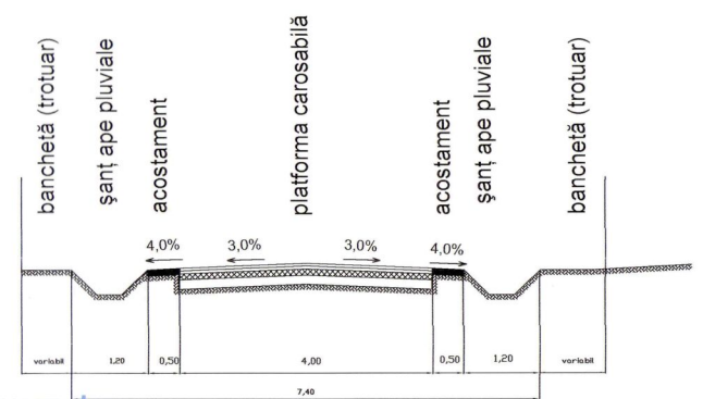
Secțiune caracteristică strazi reabilite, 4,00 m
