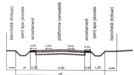
Secțiune caracteristică străzi reabilitate, 4,00 m
