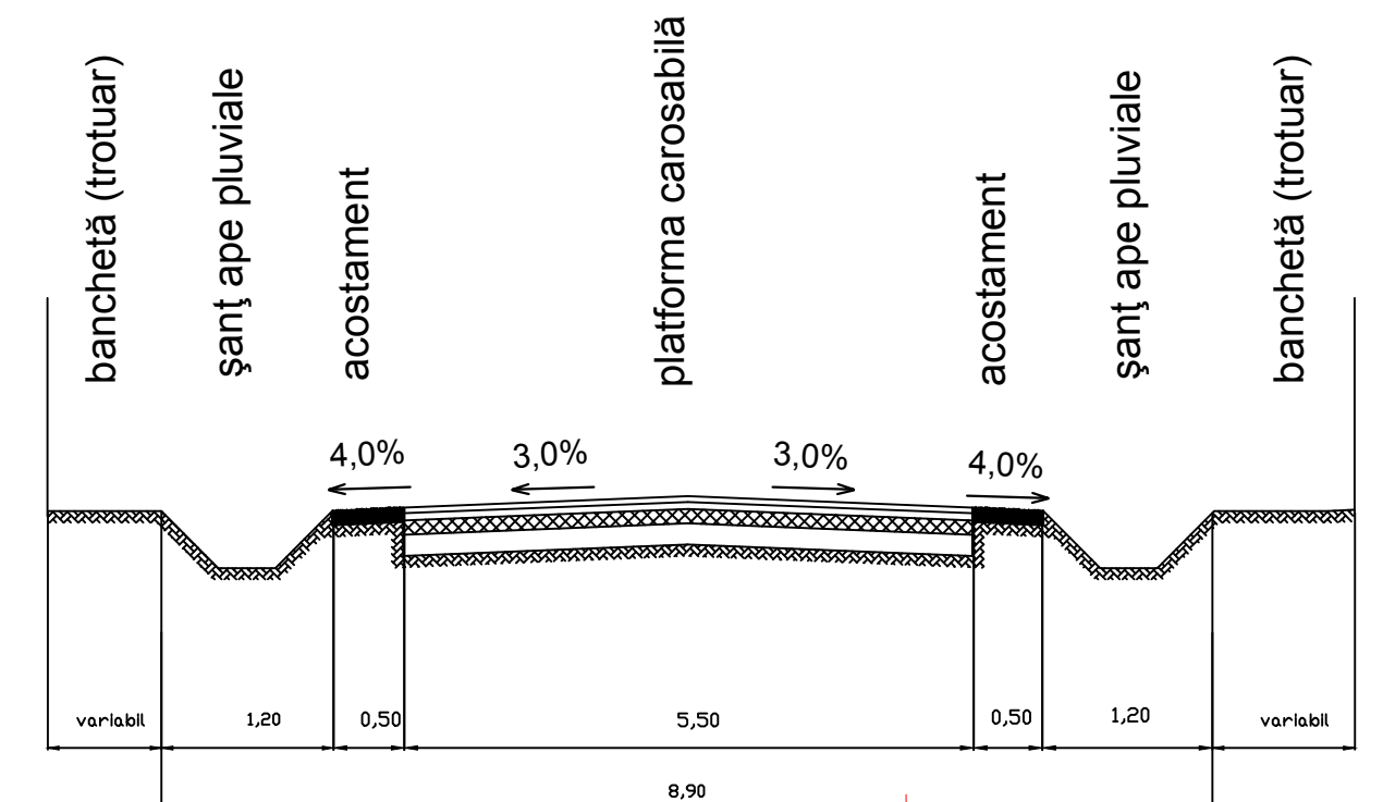
SECȚIUNE CARACTERISTICĂ STRĂZI REABILITATE, 4,00 M
